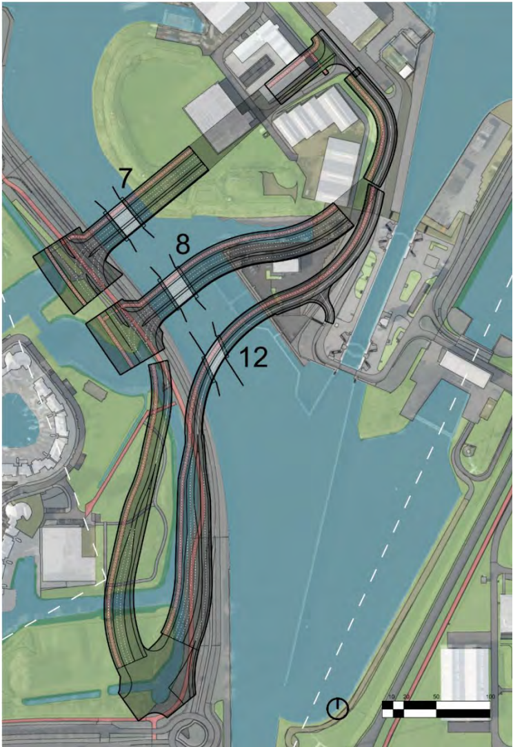
Figuur 3-9: Drie kansrijke varianten Ravelijnbrug
